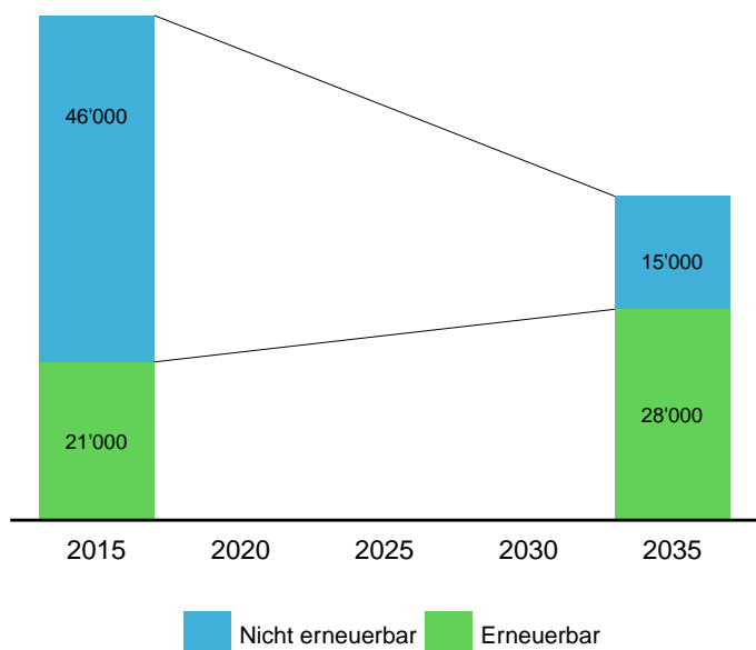
Wärmebedarf Wohngebäude: Entwicklung und Zielwerte [MWh] 3,10
