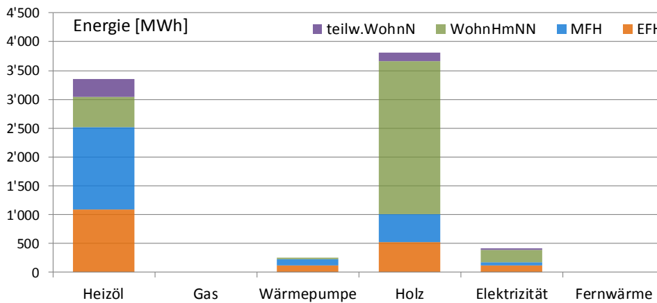
Abbildung 4: Benötigte Wärmeenergie in [MWh/a] nach Energieträger der Heizung und Gebäudekategorie. Illustration der Tabelle 7. Auszug GWR: 29. Mai 2015. Ufhusen.
