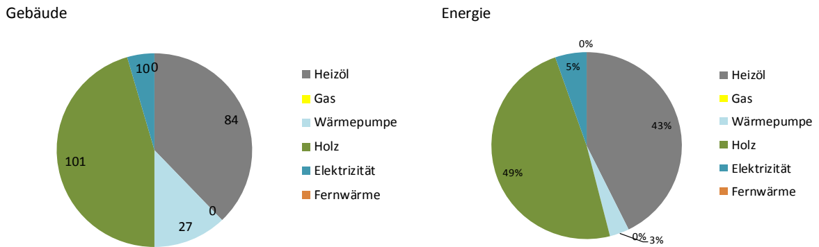
Abbildung 5: Anteile der Energieträger der Heizung nach Anzahl Gebäude und nach Anteil des Beitrages an der Wärmeenergie: Auszug GWR: 29. Mai 2015. Ufhusen.
