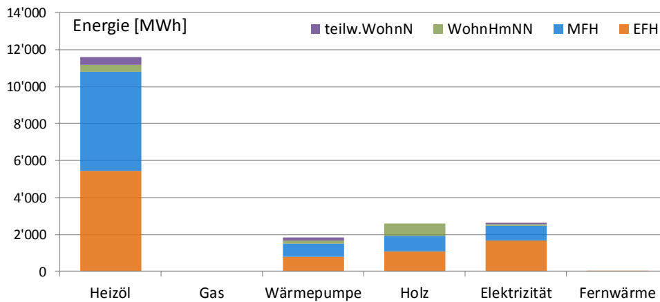
Abbildung 4: Benötigte Wärmeenergie in [MWh/a] nach Energieträger der Heizung und Gebäudekategorie. Illustration der Tabelle 7. Auszug GWR: 29. Mai 2015. Udligenswil.
