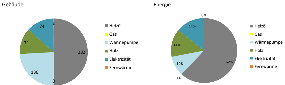
Abbildung 5: Anteile der Energieträger der Heizung nach Anzahl Gebäude und nach Anteil des Beitrages an der Wärmeenergie: Auszug GWR: 29. Mai 2015. Udligenswil.
