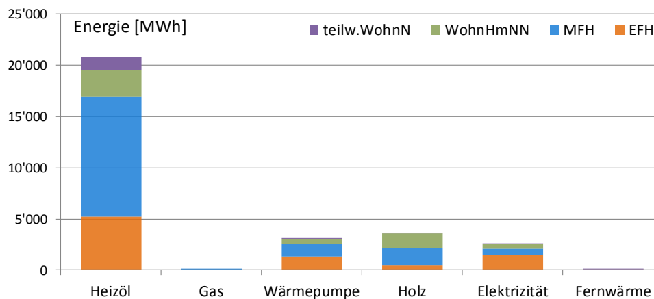
Abbildung 4: Benötigte Wärmeenergie in [MWh/a] nach Energieträger der Heizung und Gebäudekategorie. Illustration der Tabelle 7. Auszug GWR: 29. Mai 2015. Sempach.
