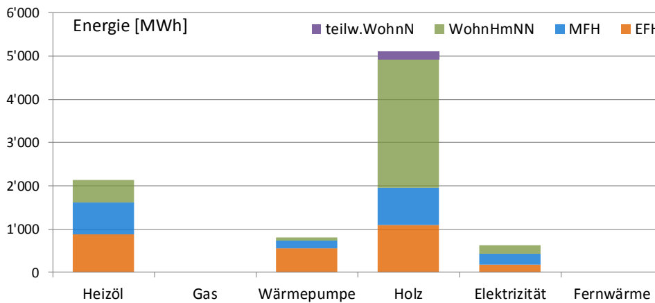
Abbildung 4: Benötigte Wärmeenergie in [MWh/a] nach Energieträger der Heizung und Gebäudekategorie. Illustration der Tabelle 7. Auszug GWR: 29. Mai 2015. Schongau.
