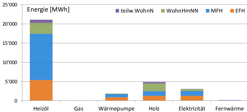
Abbildung 4: Benötigte Wärmeenergie in [MWh/a] nach Energieträger der Heizung und Gebäudekategorie. Illustration der Tabelle 7. Auszug GWR: 29. Mai 2015. Schötz.
