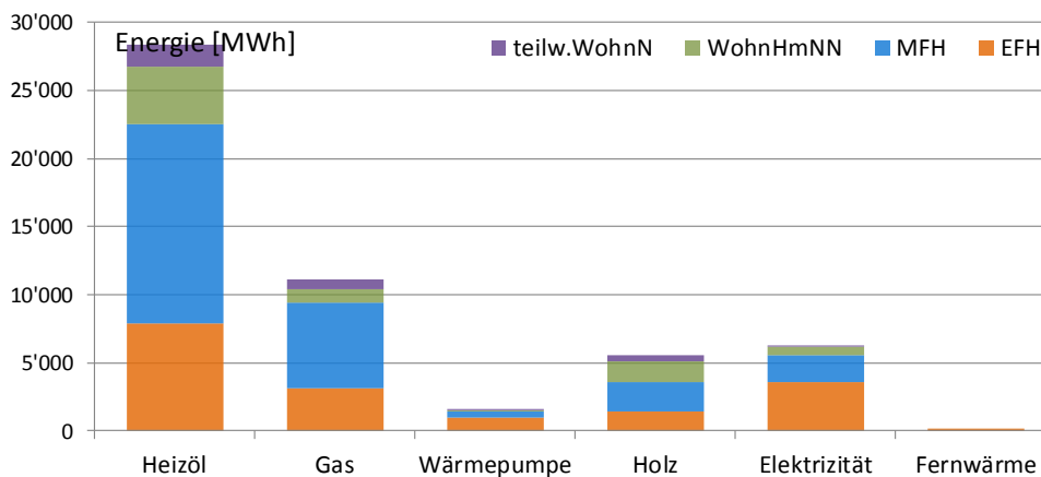
Abbildung 4: Benötigte Wärmeenergie in [MWh/a] nach Energieträger der Heizung und Gebäudekategorie. Illustration der Tabelle 7. Auszug GWR: 29. Mai 2015. Rothenburg.
