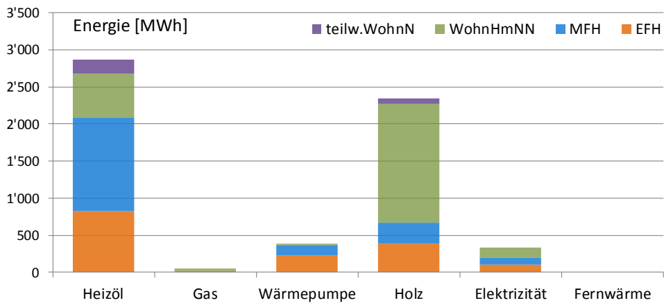
Abbildung 4: Benötigte Wärmeenergie in [MWh/a] nach Energieträger der Heizung und Gebäudekategorie. Illustration der Tabelle 7. Auszug GWR: 29. Mai 2015. Roggliswil.
