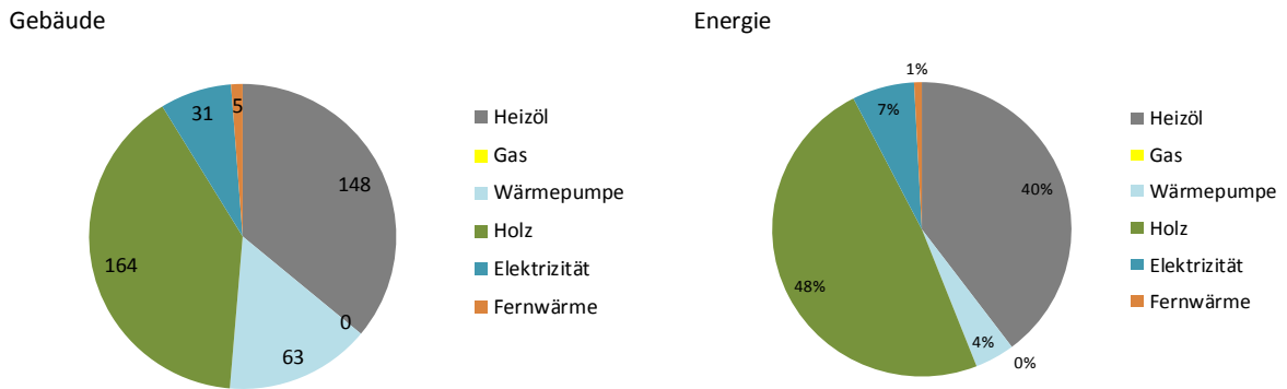
Abbildung 5: Anteile der Energieträger der Heizung nach Anzahl Gebäude und nach Anteil des Beitrages an der Wärmeenergie: Auszug GWR: 29. Mai 2015. Römerswil.
