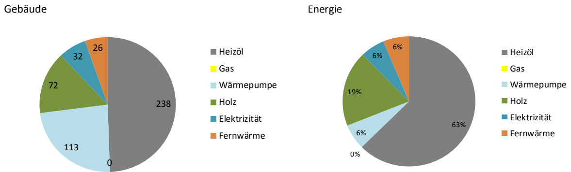
Abbildung 5: Anteile der Energieträger der Heizung nach Anzahl Gebäude und nach Anteil des Beitrages an der Wärmeenergie: Auszug GWR: 29. Mai 2015. Rain.
