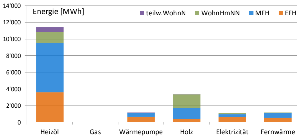
Abbildung 4: Benötigte Wärmeenergie in [MWh/a] nach Energieträger der Heizung und Gebäudekategorie. Illustration der Tabelle 7. Auszug GWR: 29. Mai 2015. Rain.
