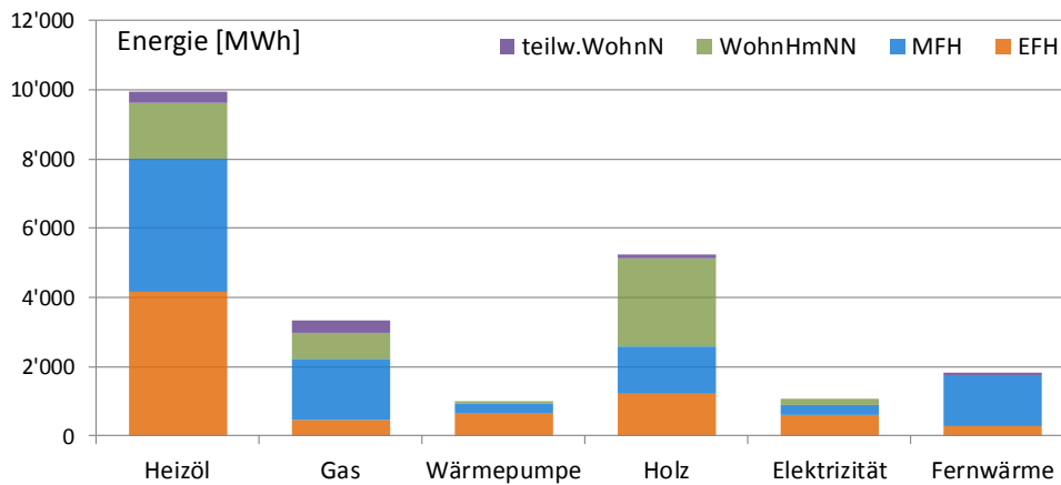
Abbildung 4: Benötigte Wärmeenergie in [MWh/a] nach Energieträger der Heizung und Gebäudekategorie. Illustration der Tabelle 7. Auszug GWR: 29. Mai 2015. Pfaffnau.
