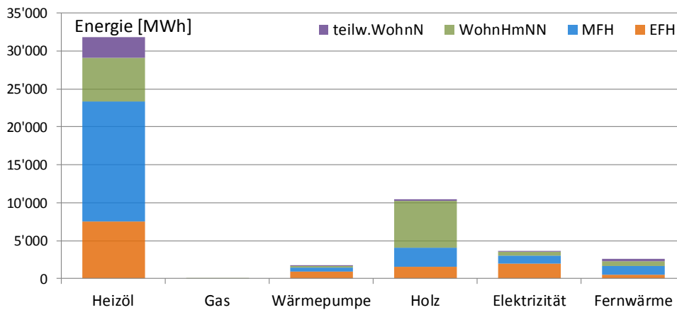
Abbildung 4: Benötigte Wärmeenergie in [MWh/a] nach Energieträger der Heizung und Gebäudekategorie. Illustration der Tabelle 7. Auszug GWR: 29. Mai 2015. Neuenkirch.
