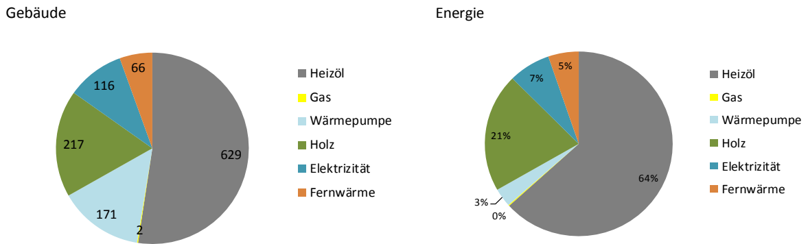
Abbildung 5: Anteile der Energieträger der Heizung nach Anzahl Gebäude und nach Anteil des Beitrages an der Wärmeenergie: Auszug GWR: 29. Mai 2015. Neuenkirch.
