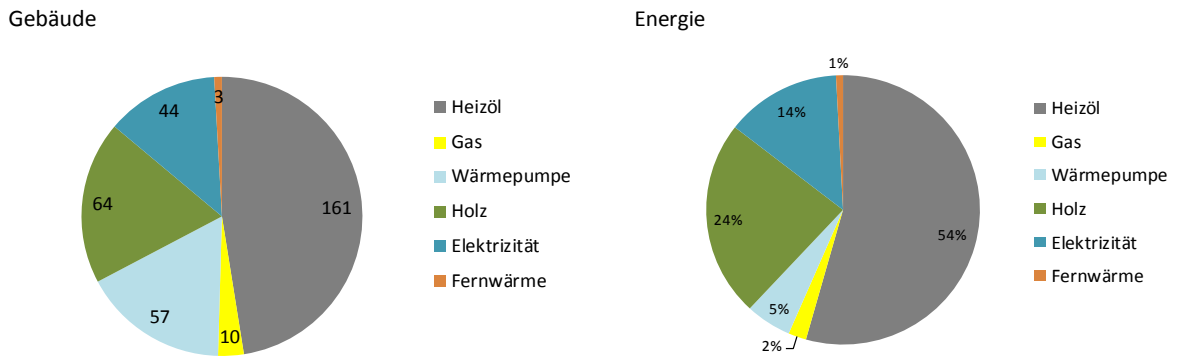
Abbildung 5: Anteile der Energieträger der Heizung nach Anzahl Gebäude und nach Anteil des Beitrages an der Wärmeenergie: Auszug GWR: 29. Mai 2015. Meierskappel.
