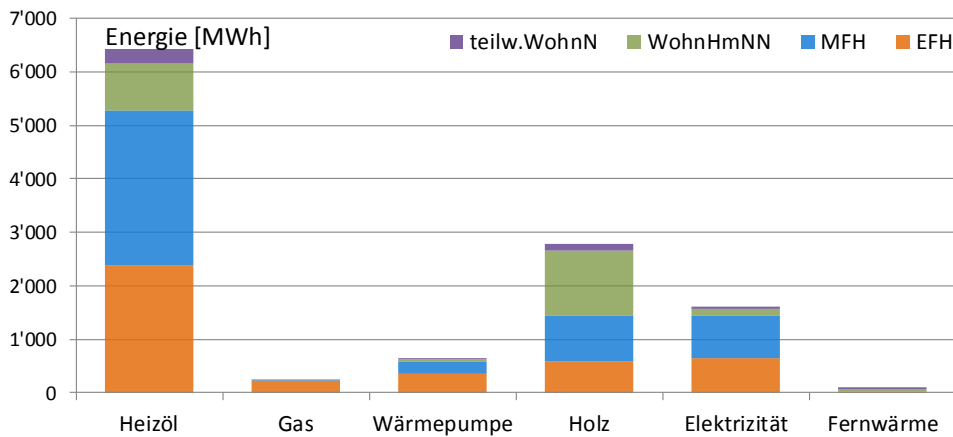
Abbildung 4: Benötigte Wärmeenergie in [MWh/a] nach Energieträger der Heizung und Gebäudekategorie. Illustration der Tabelle 7. Auszug GWR: 29. Mai 2015. Meierskappel.
