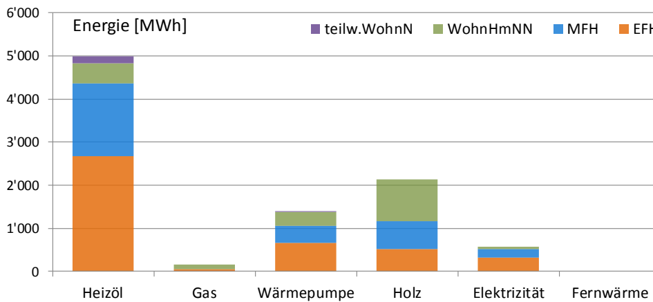
Abbildung 4: Benötigte Wärmeenergie in [MWh/a] nach Energieträger der Heizung und Gebäudekategorie. Illustration der Tabelle 7. Auszug GWR: 29. Mai 2015. Mauensee.
