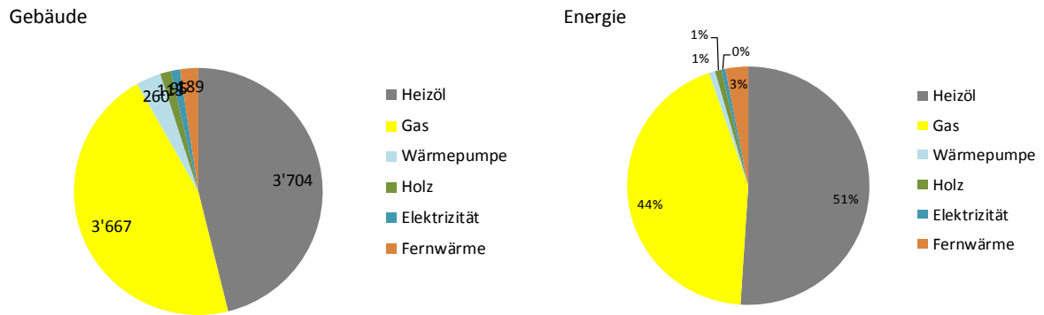
Abbildung 5: Anteile der Energieträger der Heizung nach Anzahl Gebäude und nach Anteil des Beitrages an der Wärmeenergie: Auszug GWR: 29. Mai 2015. Luzern.
