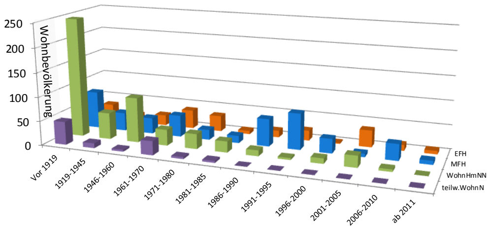
Abbildung 3: Ständige Wohnbevölkerung in der Gemeinde Luthern nach Gebäude-Kategorie und Gebäude-Baujahr. (Grafische Darstellung der Tabelle 1.) Auszug GWR per Ende 2013 durch LUSTAT Luzern Statistik.
