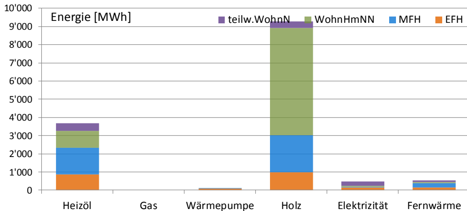
Abbildung 4: Benötigte Wärmeenergie in [MWh/a] nach Energieträger der Heizung und Gebäudekategorie. Illustration der Tabelle 7. Auszug GWR: 29. Mai 2015. Luthern.
