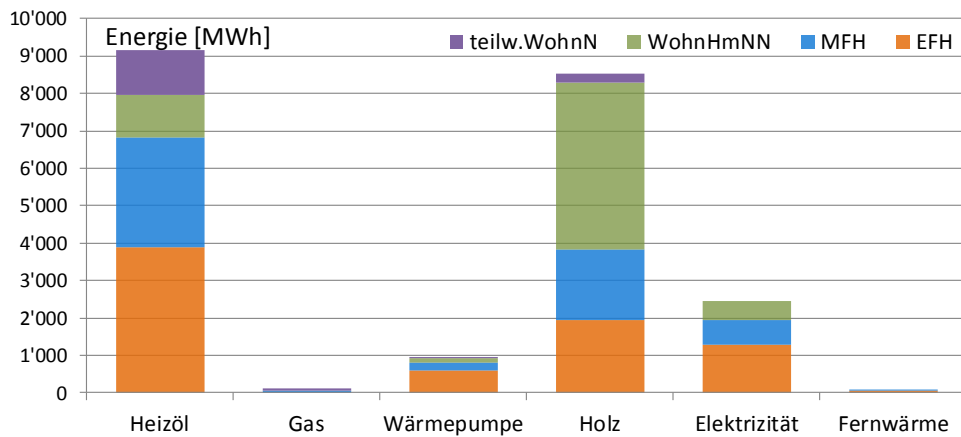
Abbildung 4: Benötigte Wärmeenergie in [MWh/a] nach Energieträger der Heizung und Gebäudekategorie. Illustration der Tabelle 7. Auszug GWR: 29. Mai 2015. Hohenrain.
