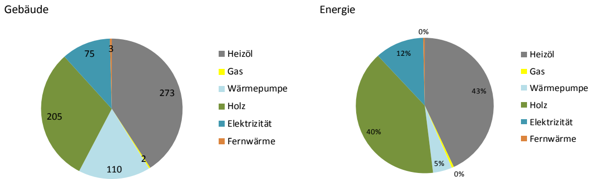
Abbildung 5: Anteile der Energieträger der Heizung nach Anzahl Gebäude und nach Anteil des Beitrages an der Wärmeenergie: Auszug GWR: 29. Mai 2015. Hohenrain.
