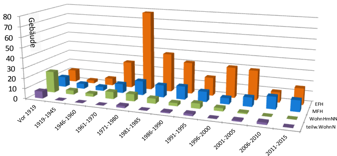
Abbildung 2: Anzahl Gebäude in der Gemeinde Hildisrieden nach Gebäude-Kategorie und Gebäude-Baujahr. Auszug GWR: 29. Mai 2015
