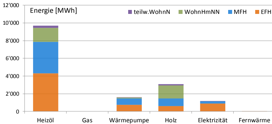
Abbildung 4: Benötigte Wärmeenergie in [MWh/a] nach Energieträger der Heizung und Gebäudekategorie. Illustration der Tabelle 7. Auszug GWR: 29. Mai 2015. Hildisrieden.
