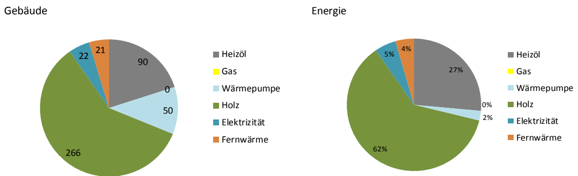
Abbildung 5: Anteile der Energieträger der Heizung nach Anzahl Gebäude und nach Anteil des Beitrages an der Wärmeenergie: Auszug GWR: 29. Mai 2015. Hergiswil bei Willisau.
