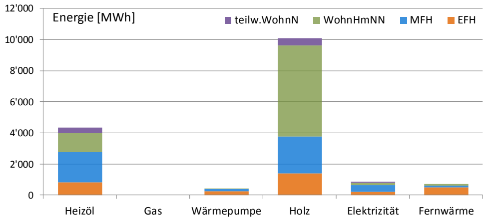
Abbildung 4: Benötigte Wärmeenergie in [MWh/a] nach Energieträger der Heizung und Gebäudekategorie. Illustration der Tabelle 7. Auszug GWR: 29. Mai 2015. Hergiswil bei Willisau.
