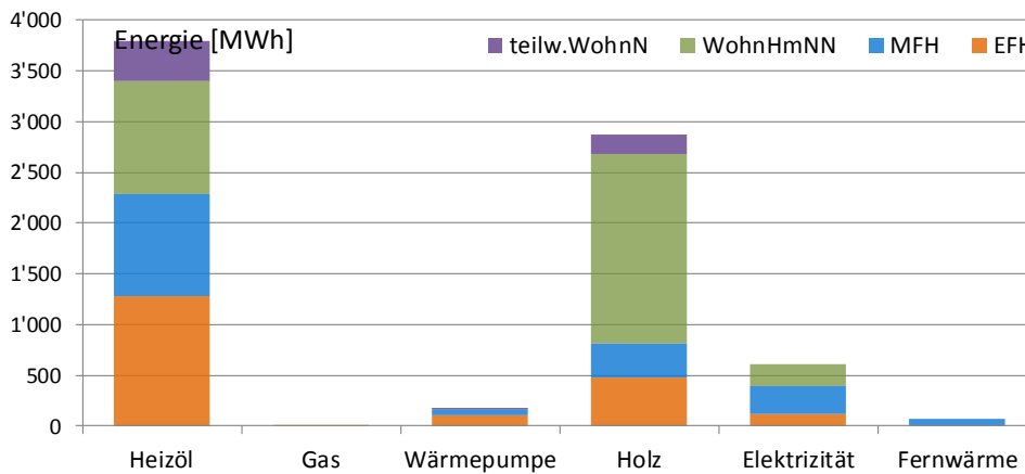
Abbildung 4: Benötigte Wärmeenergie in [MWh/a] nach Energieträger der Heizung und Gebäudekategorie. Illustration der Tabelle 7. Auszug GWR: 29. Mai 2015. Grossdietwil.
