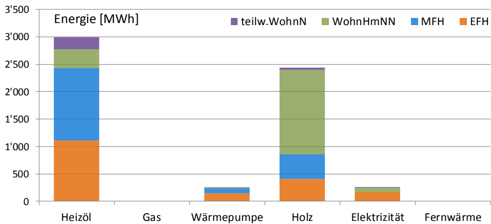
Abbildung 4: Benötigte Wärmeenergie in [MWh/a] nach Energieträger der Heizung und Gebäudekategorie. Illustration der Tabelle 7. Auszug GWR: 29. Mai 2015. Fischbach.
