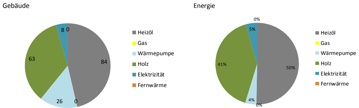
Abbildung 5: Anteile der Energieträger der Heizung nach Anzahl Gebäude und nach Anteil des Beitrages an der Wärmeenergie: Auszug GWR: 29. Mai 2015. Fischbach.
