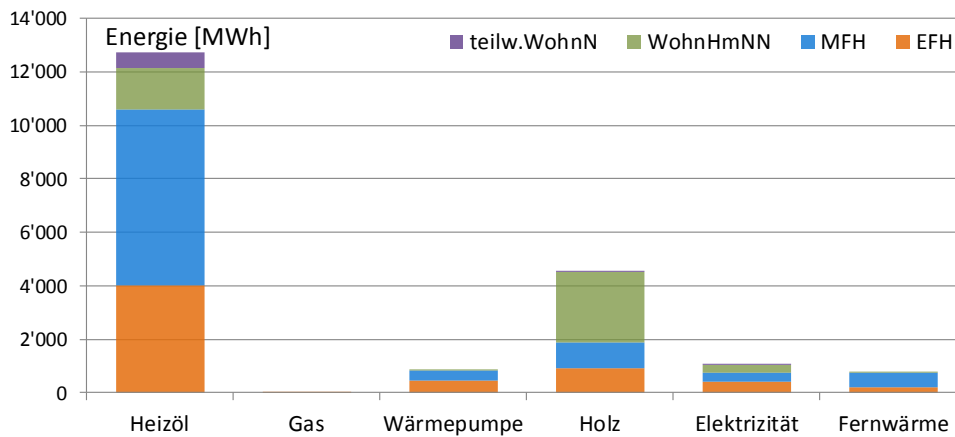
Abbildung 4: Benötigte Wärmeenergie in [MWh/a] nach Energieträger der Heizung und Gebäudekategorie. Illustration der Tabelle 7. Auszug GWR: 29. Mai 2015. Ettiswil.
