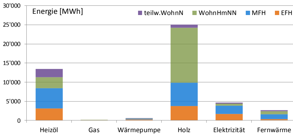
Abbildung 4: Benötigte Wärmeenergie in [MWh/a] nach Energieträger der Heizung und Gebäudekategorie. Illustration der Tabelle 7. Auszug GWR: 29. Mai 2015. Escholzmatt-Marbach.
