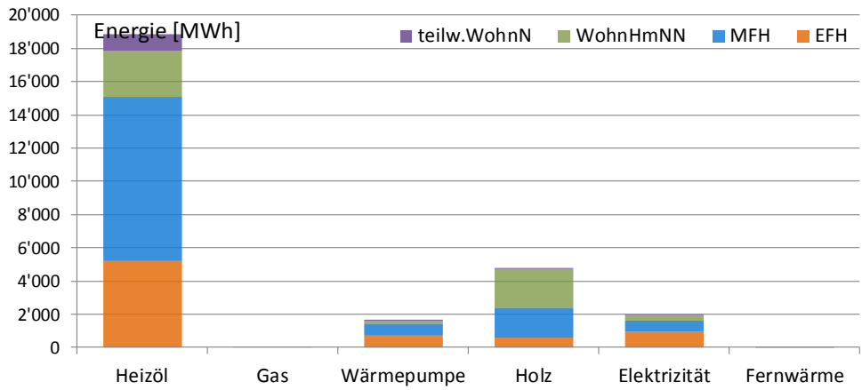
Abbildung 4: Benötigte Wärmeenergie in [MWh/a] nach Energieträger der Heizung und Gebäudekategorie. Illustration der Tabelle 7. Auszug GWR: 29. Mai 2015. Eschenbach (LU).
