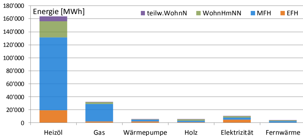
Abbildung 4: Benötigte Wärmeenergie in [MWh/a] nach Energieträger der Heizung und Gebäudekategorie. Illustration der Tabelle 7. Auszug GWR: 29. Mai 2015. Emmen.
