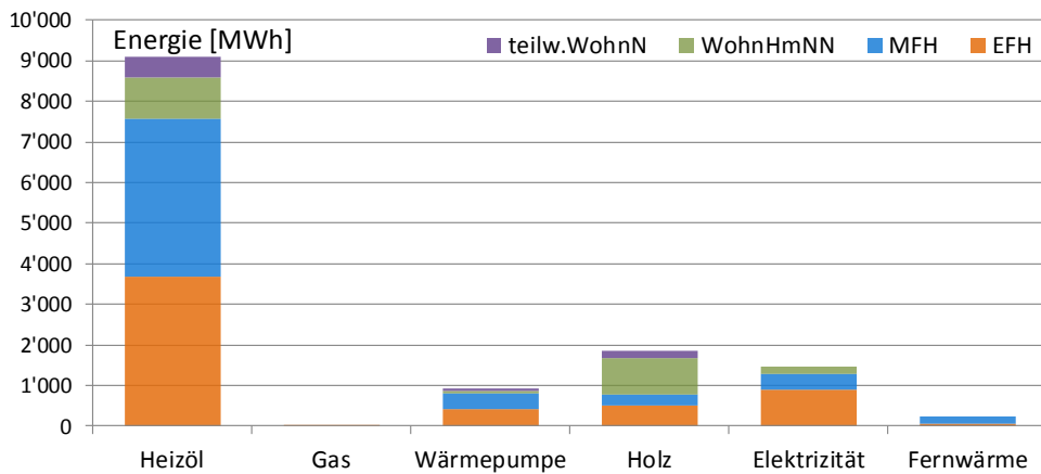
Abbildung 4: Benötigte Wärmeenergie in [MWh/a] nach Energieträger der Heizung und Gebäudekategorie. Illustration der Tabelle 7. Auszug GWR: 29. Mai 2015. Eich.
