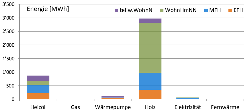
Abbildung 4: Benötigte Wärmeenergie in [MWh/a] nach Energieträger der Heizung und Gebäudekategorie. Illustration der Tabelle 7. Auszug GWR: 29. Mai 2015. Ebersecken.
