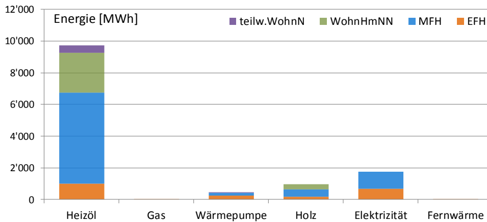
Abbildung 4: Benötigte Wärmeenergie in [MWh/a] nach Energieträger der Heizung und Gebäudekategorie. Illustration der Tabelle 7. Auszug GWR: 29. Mai 2015. Dierikon.
