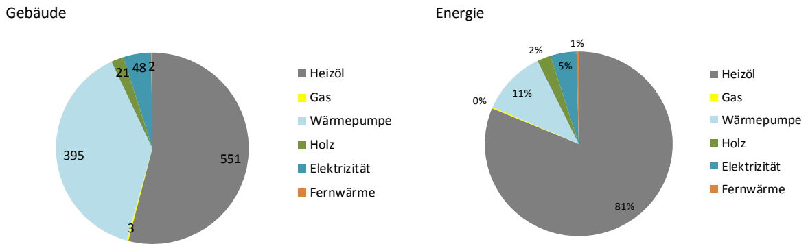
Abbildung 5: Anteile der Energieträger der Heizung nach Anzahl Gebäude und nach Anteil des Beitrages an der Wärmeenergie: Auszug GWR: 29. Mai 2015. Buchrain.
