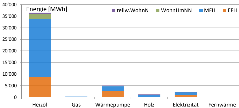
Abbildung 4: Benötigte Wärmeenergie in [MWh/a] nach Energieträger der Heizung und Gebäudekategorie. Illustration der Tabelle 7. Auszug GWR: 29. Mai 2015. Buchrain.
