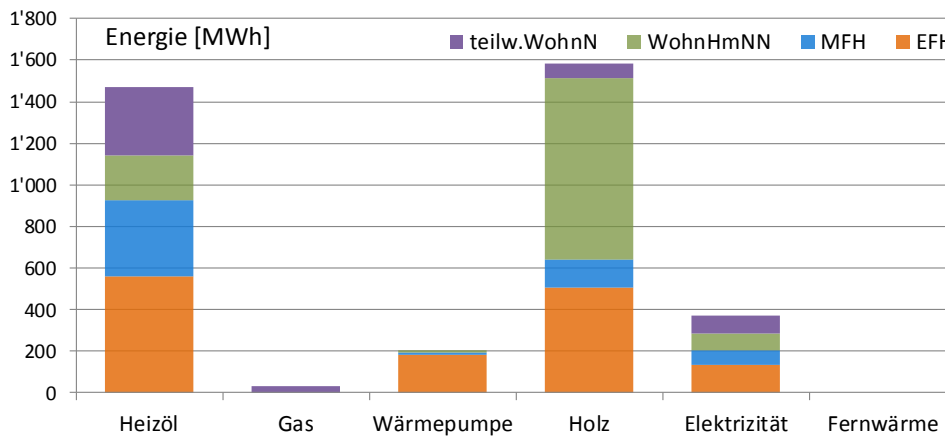
Abbildung 4: Benötigte Wärmeenergie in [MWh/a] nach Energieträger der Heizung und Gebäudekategorie. Illustration der Tabelle 7. Auszug GWR: 29. Mai 2015. Altwis.
