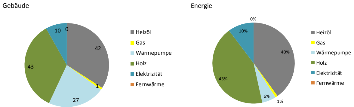
Abbildung 5: Anteile der Energieträger der Heizung nach Anzahl Gebäude und nach Anteil des Beitrages an der Wärmeenergie: Auszug GWR: 29. Mai 2015. Altwis.
