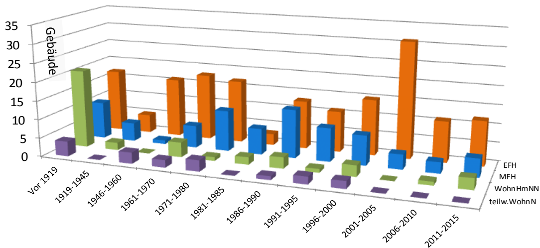
Abbildung 2: Anzahl Gebäude in der Gemeinde Altishofen nach Gebäude-Kategorie und Gebäude-Baujahr. Auszug GWR: 29. Mai 2015
