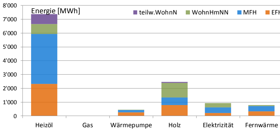
Abbildung 4: Benötigte Wärmeenergie in [MWh/a] nach Energieträger der Heizung und Gebäudekategorie. Illustration der Tabelle 7. Auszug GWR: 29. Mai 2015. Altishofen.
