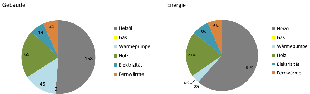
Abbildung 5: Anteile der Energieträger der Heizung nach Anzahl Gebäude und nach Anteil des Beitrages an der Wärmeenergie: Auszug GWR: 29. Mai 2015. Altishofen.
