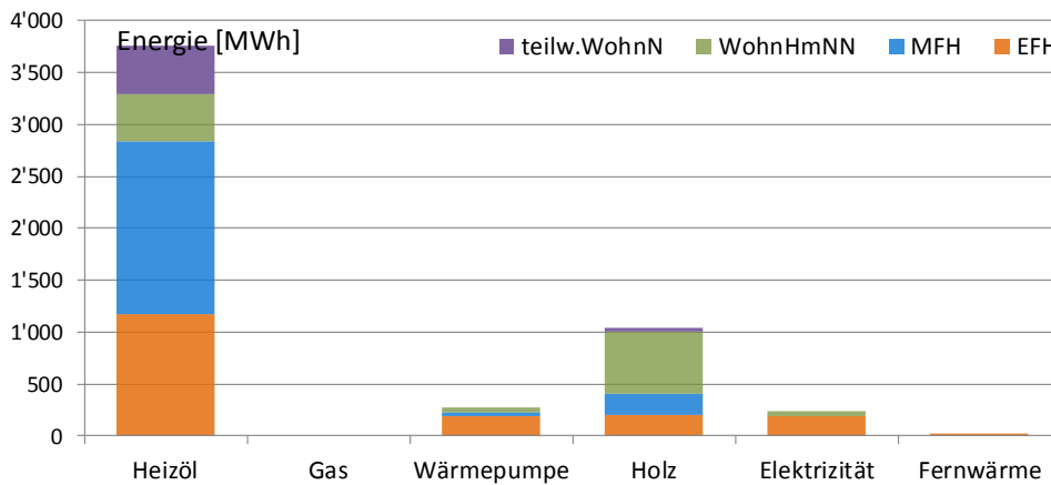
Abbildung 4: Benötigte Wärmeenergie in [MWh/a] nach Energieträger der Heizung und Gebäudekategorie. Illustration der Tabelle 7. Auszug GWR: 29. Mai 2015. Alberswil.
