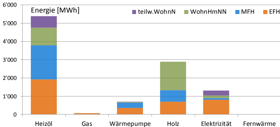
Abbildung 4: Benötigte Wärmeenergie in [MWh/a] nach Energieträger der Heizung und Gebäudekategorie. Illustration der Tabelle 7. Auszug GWR: 29. Mai 2015. Aesch (LU).
