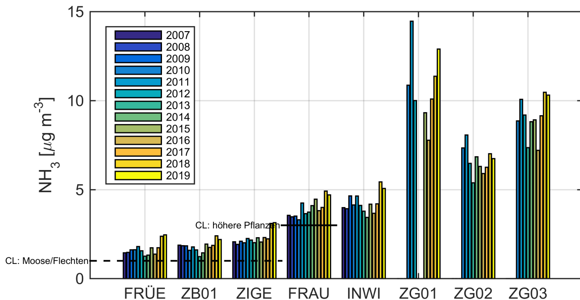
Abbildung 8: Jahresmittel (2007 bis 2019) der Ammoniakkonzentration an den einzelnen Messpunkten im Kanton Zug. Dies beinhaltet sowohl die kantonalen Messpunkte (FRÜE, ZB01, ZIGE, FRAU, INWI), wie auch diejenigen des Ressourcenprojekts (ZG0, ZG02, ZG03). Für ZG01 konnten aufgrund von Datenlücken keine gültigen Jahresmittel für 2013 und 2014 berechnet werden. Die schwarze ausgezogene Linie kennzeichnet den Critical Level (CL) für höhere Pflanzen, die schwarze gestrichelte Linie den Critical Level (CL) für empfindliche Moose und Flechten.
