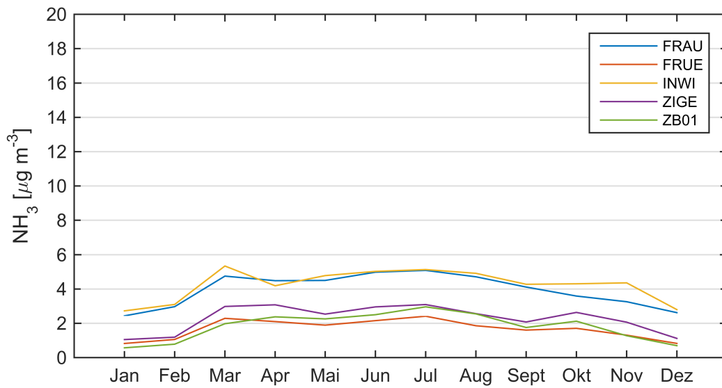
Abbildung 6: Vergleich des Jahresgangs unterschiedlicher Messpunkte mit unterschiedlicher Bewirtschaftung bzw. unterschiedlich intensiver Tierhaltung. Mittelung von 2010 bis 2019. Oben: Messpunkte von Obwalden. Unten: Messpunkte des Kantons Zug.
