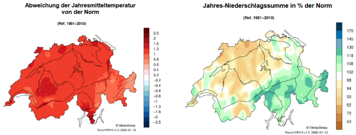
Abbildung 25: Links: Abweichung der Jahresmitteltemperatur 2019 von der Norm in °C (1981-2010). Rechts: Jahres-Niederschlagssumme in Prozent der Norm (1981-2010). Quelle: MeteoSchweiz (2020). Klimabulletin 2019.
