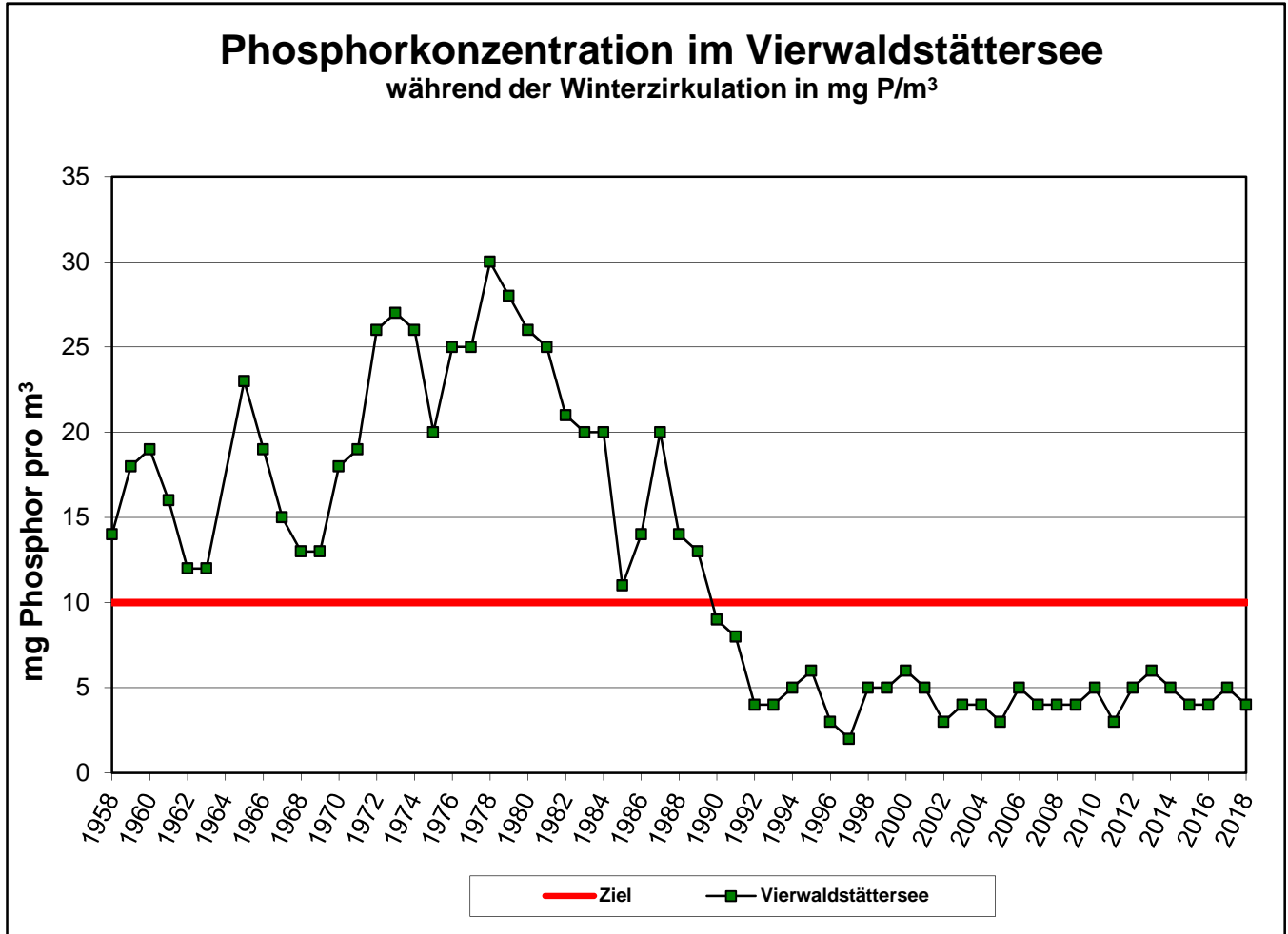
Entwicklung der Konzentration an Gesamt-Phosphor im Vierwaldstättersee von 1958 bis 2018
