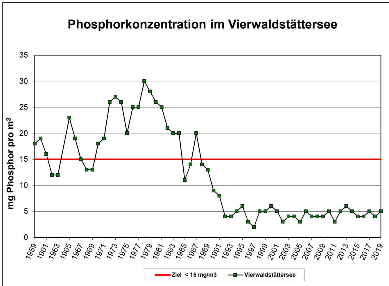
Entwicklung der Konzentration an Gesamt-Phosphor im Vierwaldstättersee von 1959 bis 2019
