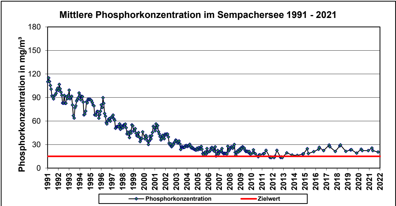
Entwicklung der Konzentration an Gesamt-Phosphor im Sempachersee von 1991 bis 2021
