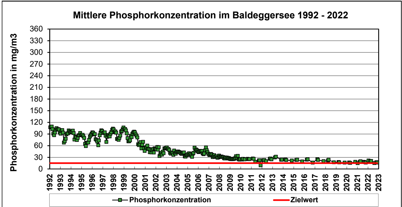
Entwicklung der Konzentration an Gesamt-Phosphor im Baldeggersee von 1992 bis 2022
