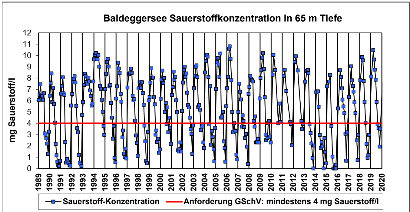
Sauerstoffgehalt im Baldeggersee am Seegrund in 65 m Tiefe
