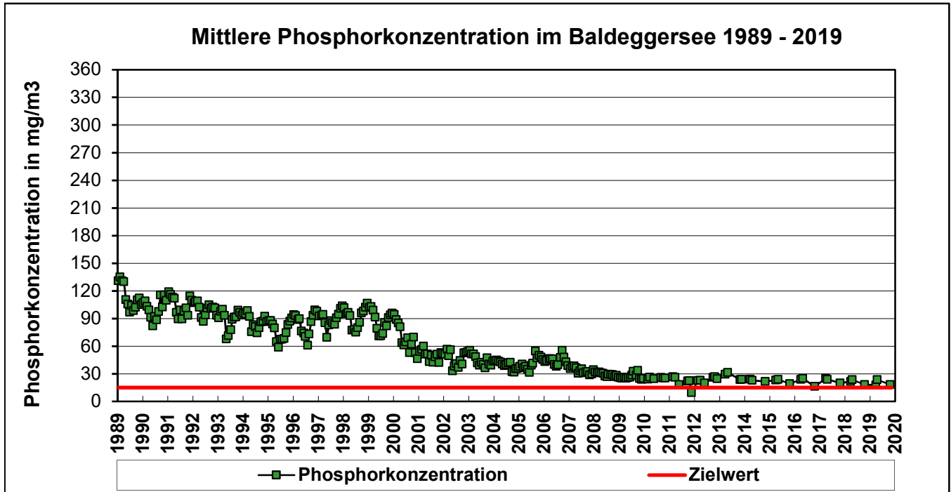
Entwicklung der Konzentration an Gesamt-Phosphor im Baldeggersee von 1989 bis 2019
